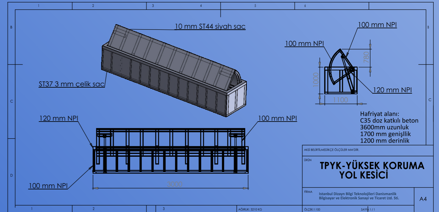
Teknik Ölçüler
